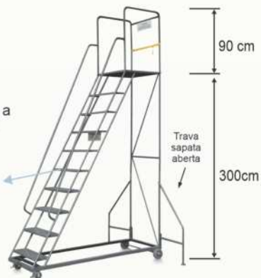
Degraus em Chapa Xadrez
