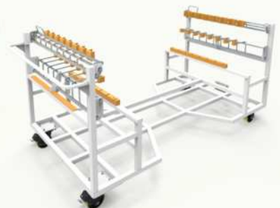
**Rack para transporte de fechamento superior central
